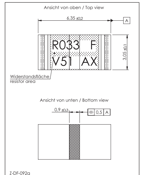
Bauform / Size 2512
