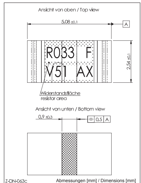
Bauform / Size 2010
